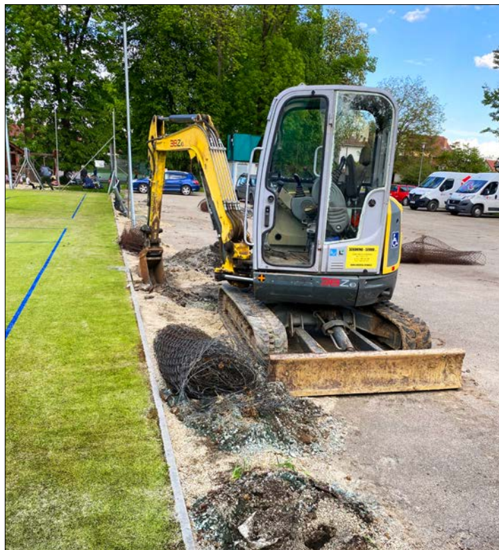
Rekonstrukce plotu na víceúčelovém hřišti u sokolovny
