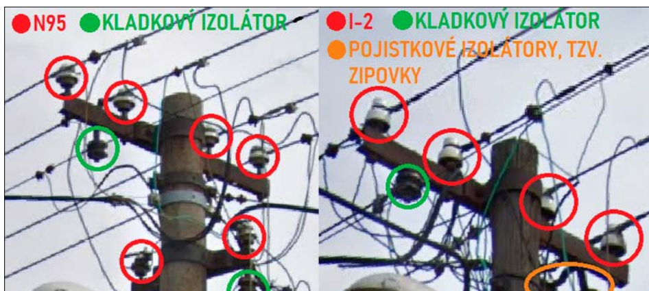
Vlevo je novější sloup, popsané izolátory N95 a kladkový izolátor. Vpravo je starší sloup, popsané izolátory I-2, kladkový izolátor a pojistkové izolátory, tzv. zipovky, které se dříve používaly místo klasických pojistek. Dříve totiž vždy nebyly pojistky na domě, ale zašroubované v izolátoru na sloupu. Pokud se chtěly pojistky měnit, muselo se vylézt na sloup.
